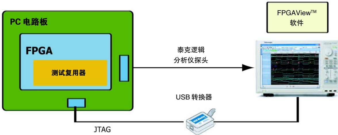
► 图 2. 典型的 FPGAView 实现方案。
