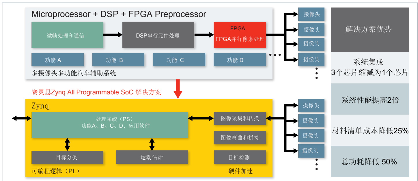
驾驶员辅助应用中，Zynq All Programmable SoC 与多芯片摄像头系统对比
